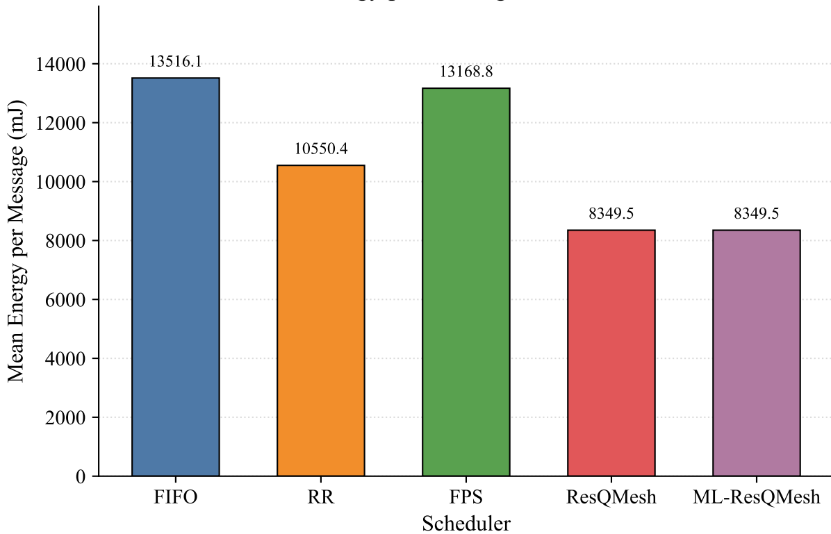
Mean Energy per Message - SOS Intensive
